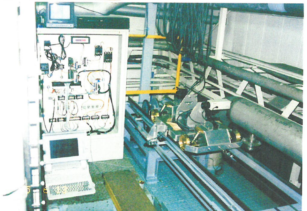
波形追従ビデオ撮影カート
